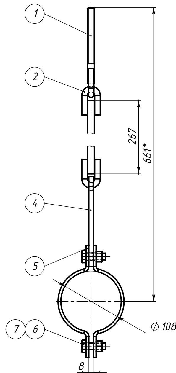
Поз.5 (Полухомут)
