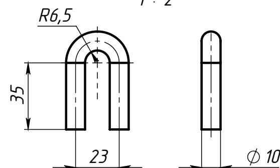
Поз.2 (Ушко) 1:2
